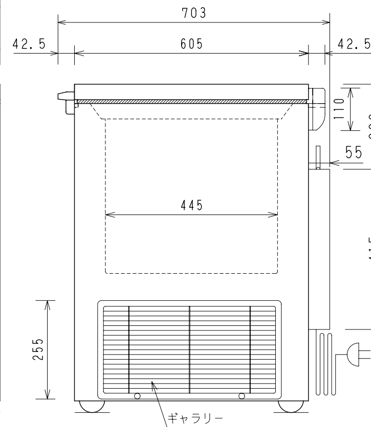
側面図
