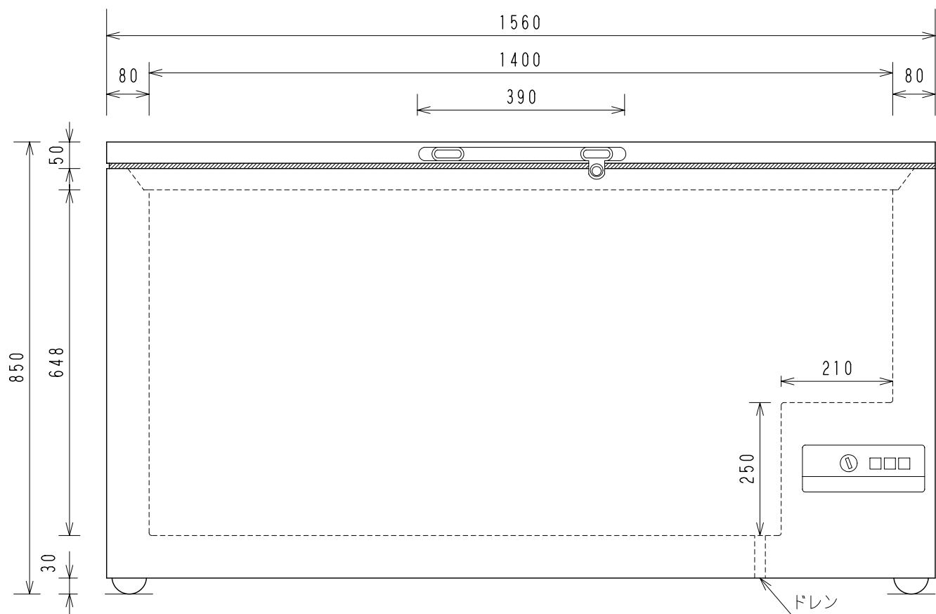
正面図
